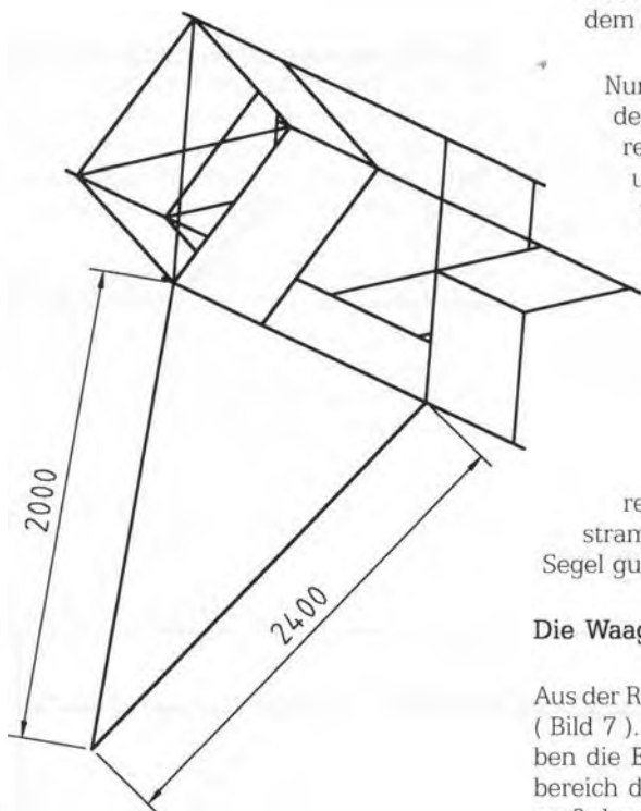
Bild 7: Gesamtansicht mit Waagenmaßen
